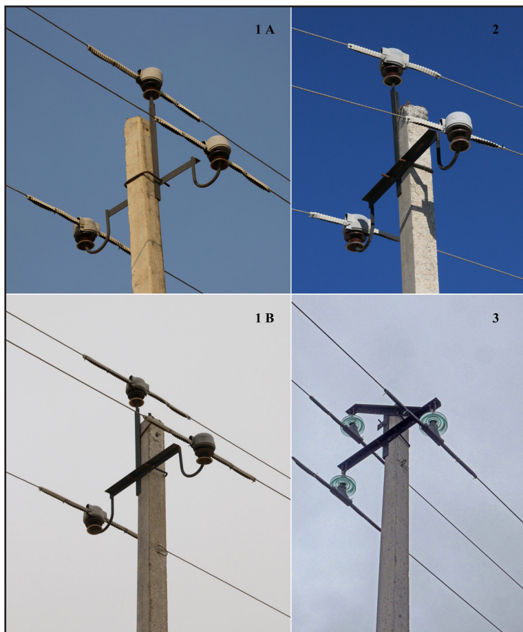
Рис. 4. ПЗУ, установленные на участке ВЛЭ АО «КазТрансГаз» в окрестностях пос. Акжигит, обеспечивают безопасность крупных птиц, т.к. снабжены достаточно длинными (двойными) рукавами, изолирующими не менее 1 м токонесущего провода вблизи изолятора – 1А, 1В; ПЗУ, установленные на участке ВЛЭ АО «КазТрансГаз» в Каракиянском районе, снабжены слишком короткими (одинарными) рукавами, изолируют лишь около 0,5 м токонесущего провода вблизи изолятора и не обеспечивают безопасность крупных птиц с размахом крыльев более 1 м – 2; траверсы «ласточкин хвост», оборудованы полимерными ПЗУ на протяжении 270 км ВЛЭ АО «Интергаз Центральная Азия» (подразделение АО «КазТрансГаз») в ходе их реконструкции в 2015 г. уже после реализации нашего проекта – 3. Фото М. Пестова и Д. Тарасова.
